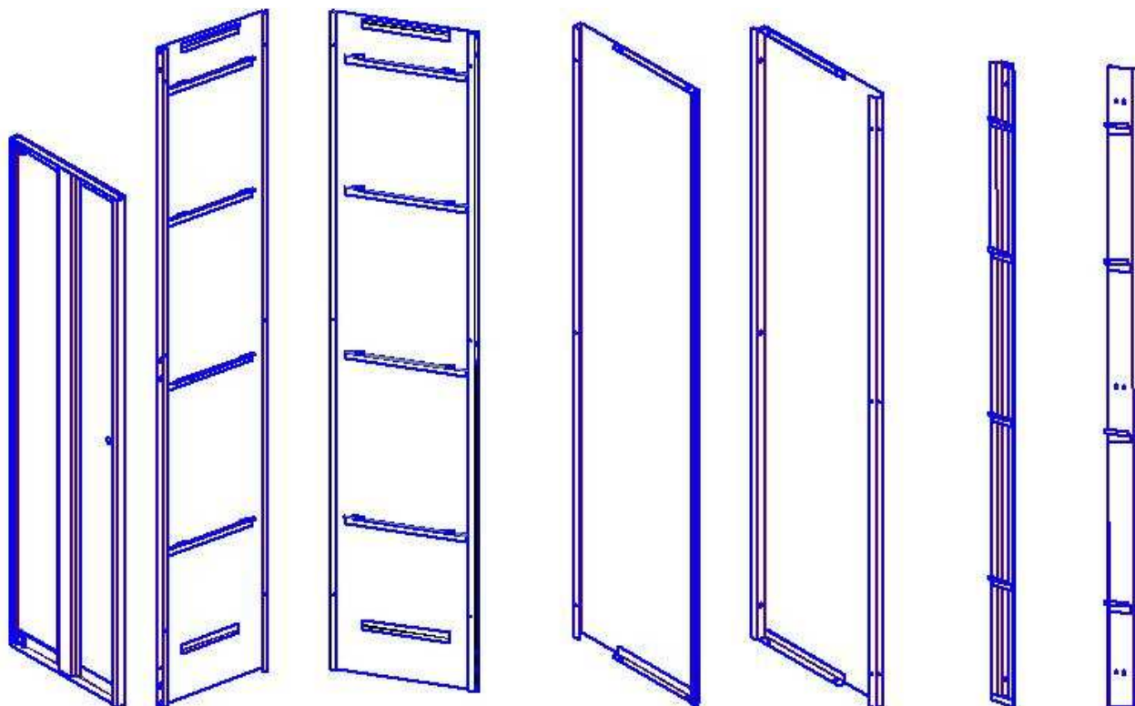
Рис. 2 Дверь
